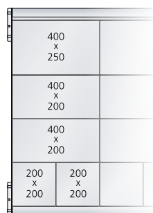
Lagerkasten-Beispielkonfigurationen bei 864 mm Tablartiefe
